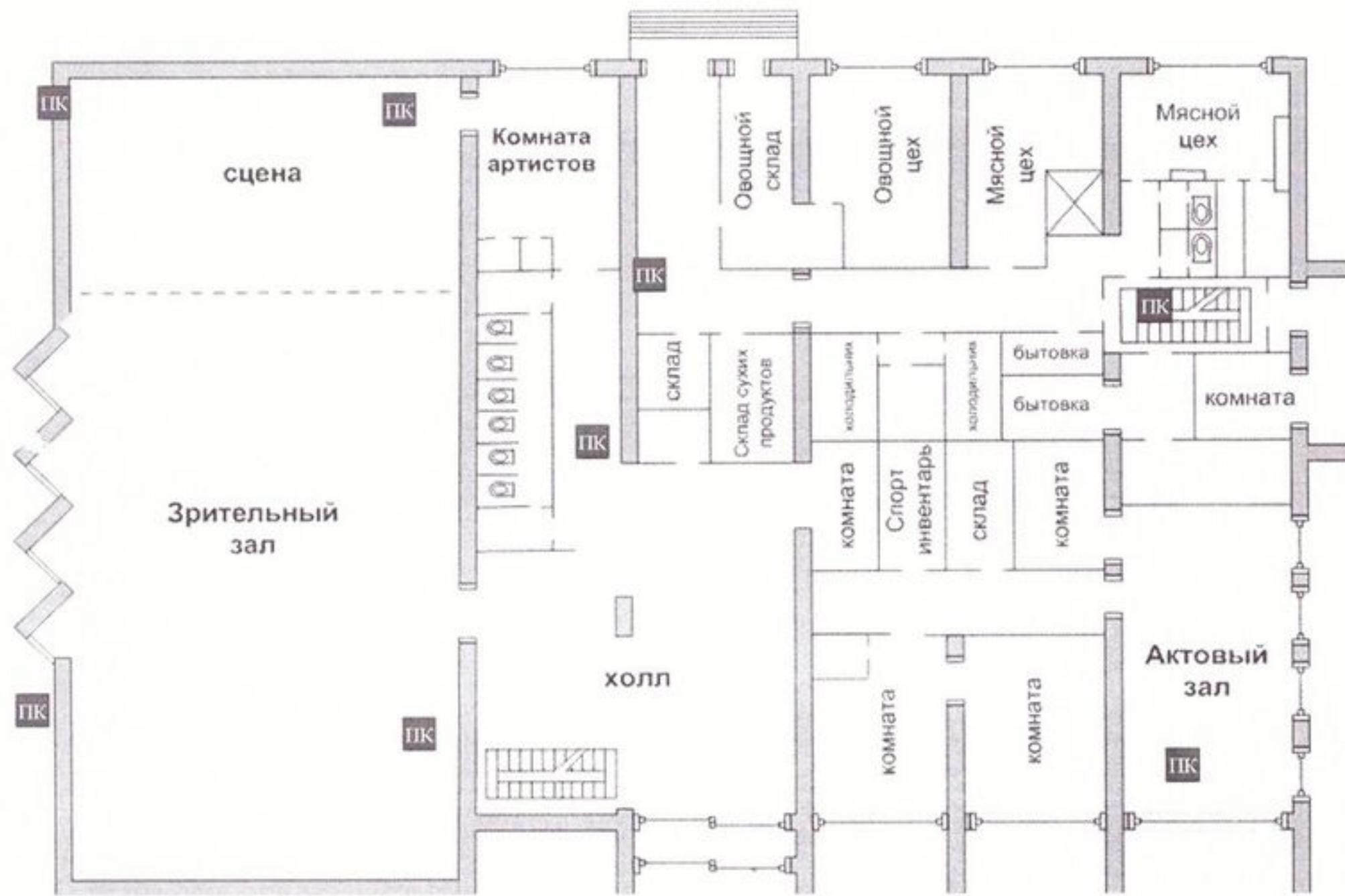
Столовая 2 этаж
